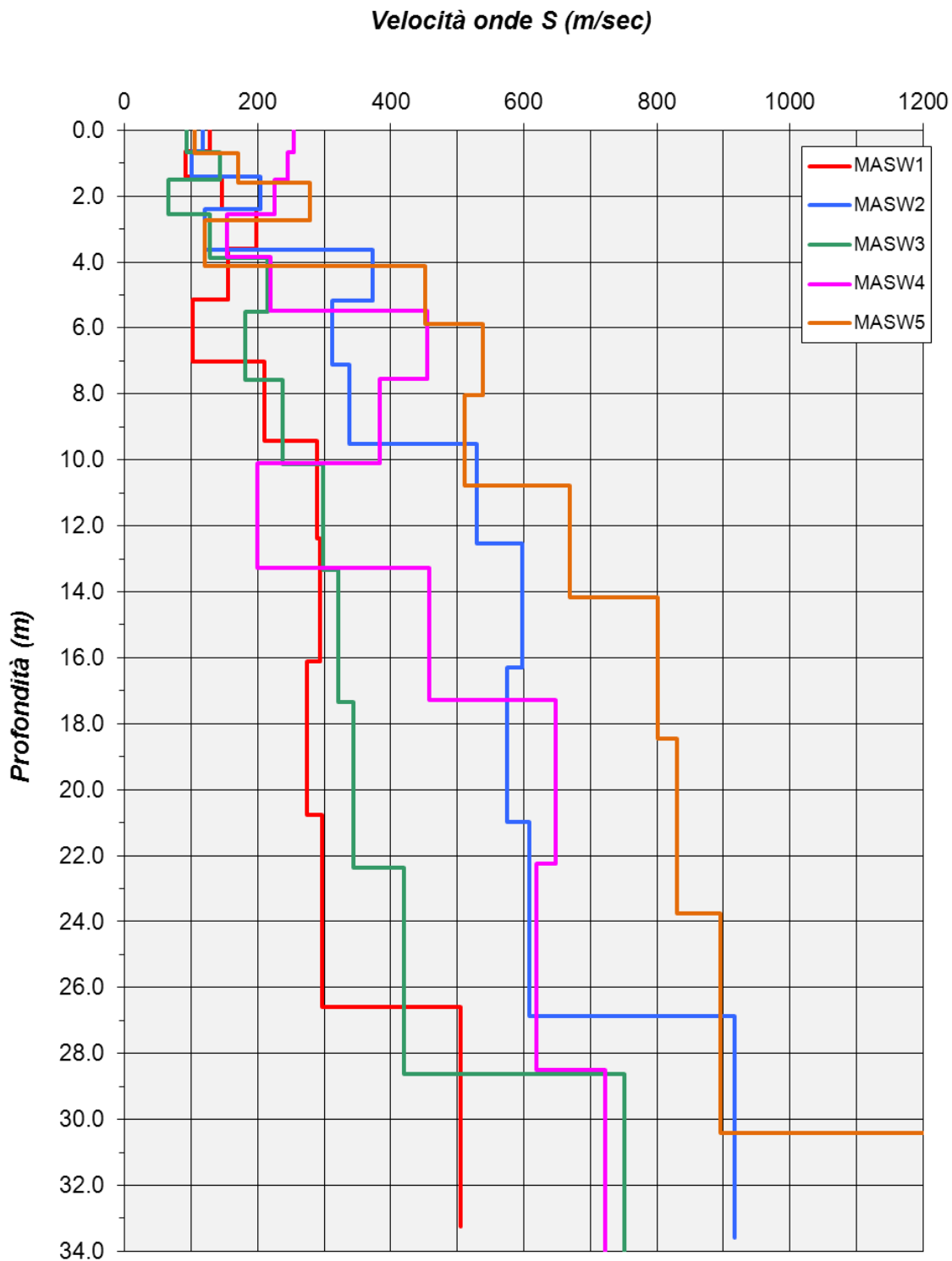
Figura 8: andamento con la profondità della velocità delle onde S per le aree indagate.
